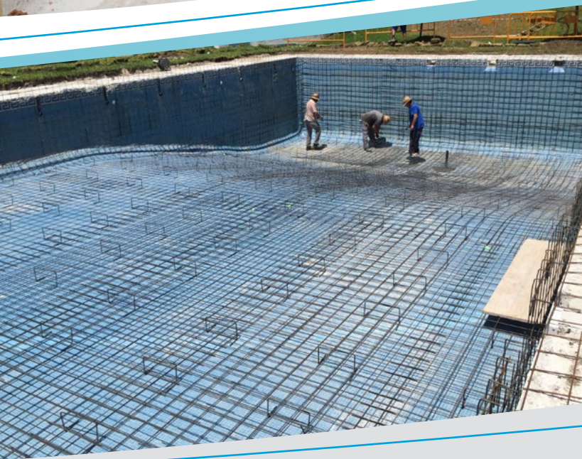
■ Colocación de nuevo mallazo en vaso piscina
